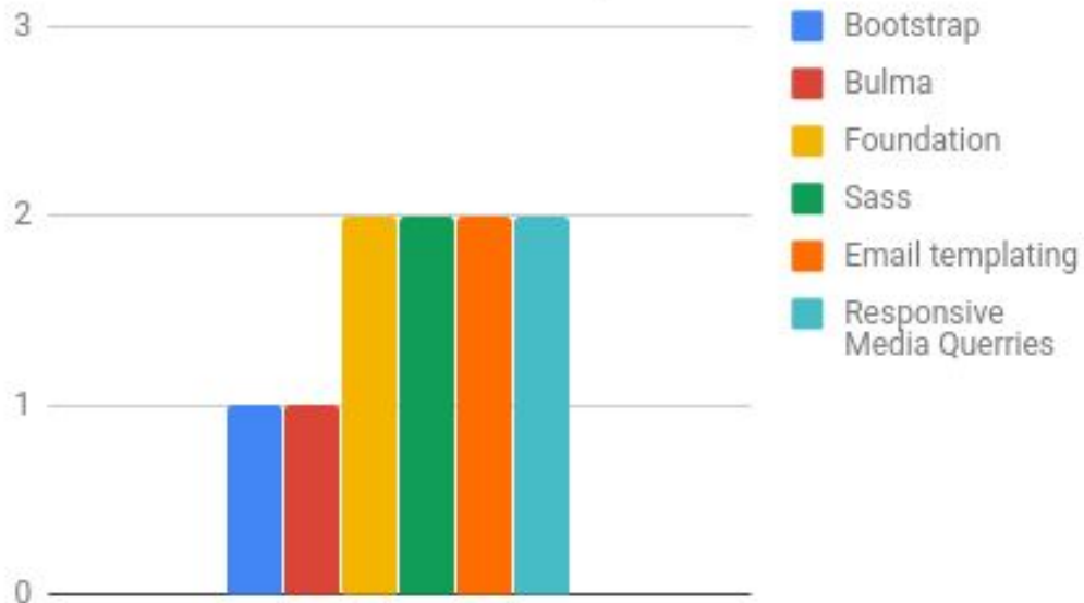
Frontend HTML/CSS
